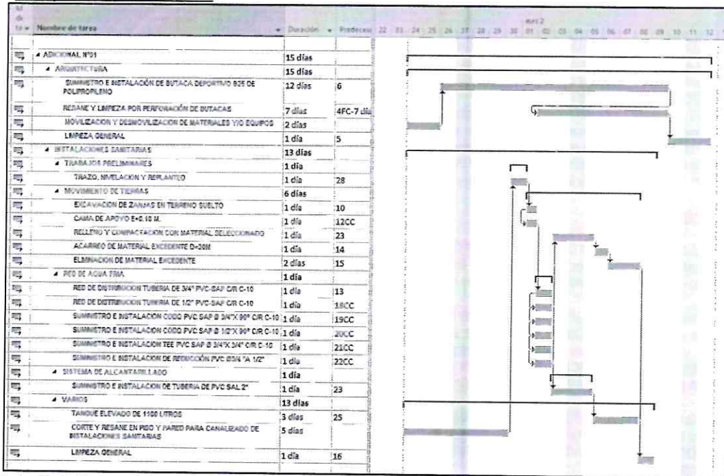
Ilustración 1: Plazo aprobado para la ejecución del adicional de obra Fuente: Expediente técnico de adicional de obra N°01
